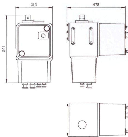
Sl. 1 Motorni pogon MP5 1 ábra MP5 motoros hajtás
