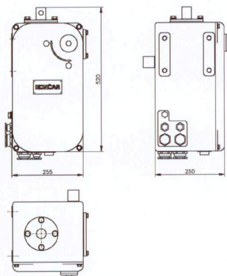
Sl. 2 Ručni pogon RP 5 2 ábra RP5 kézi hajtás
